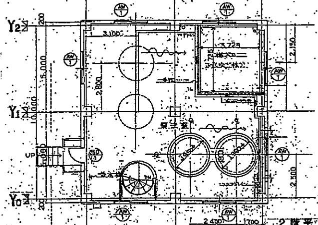
2階平面図
