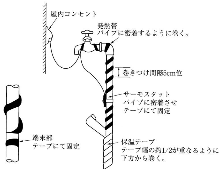
例) 凍結防止ヒーターの施工
