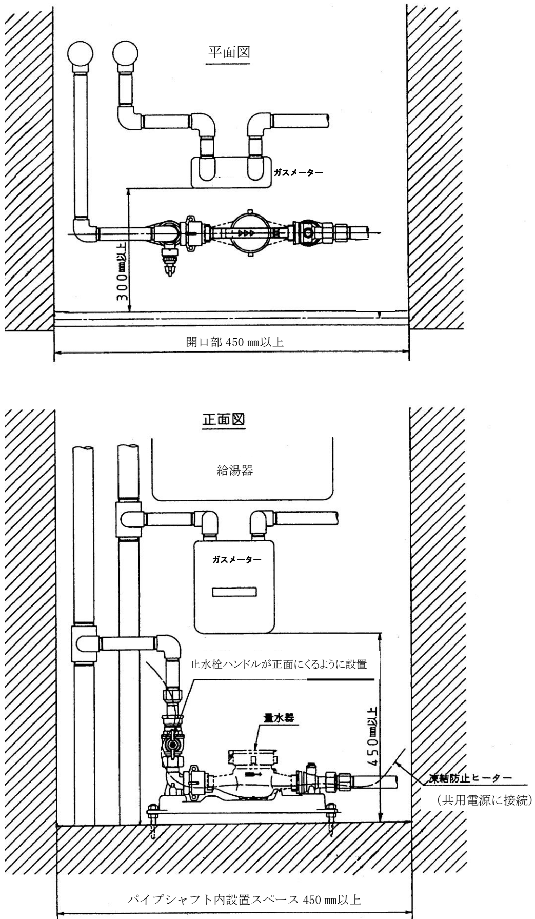
図6-4 パイプシャフト内メーターユニット標準配管図
