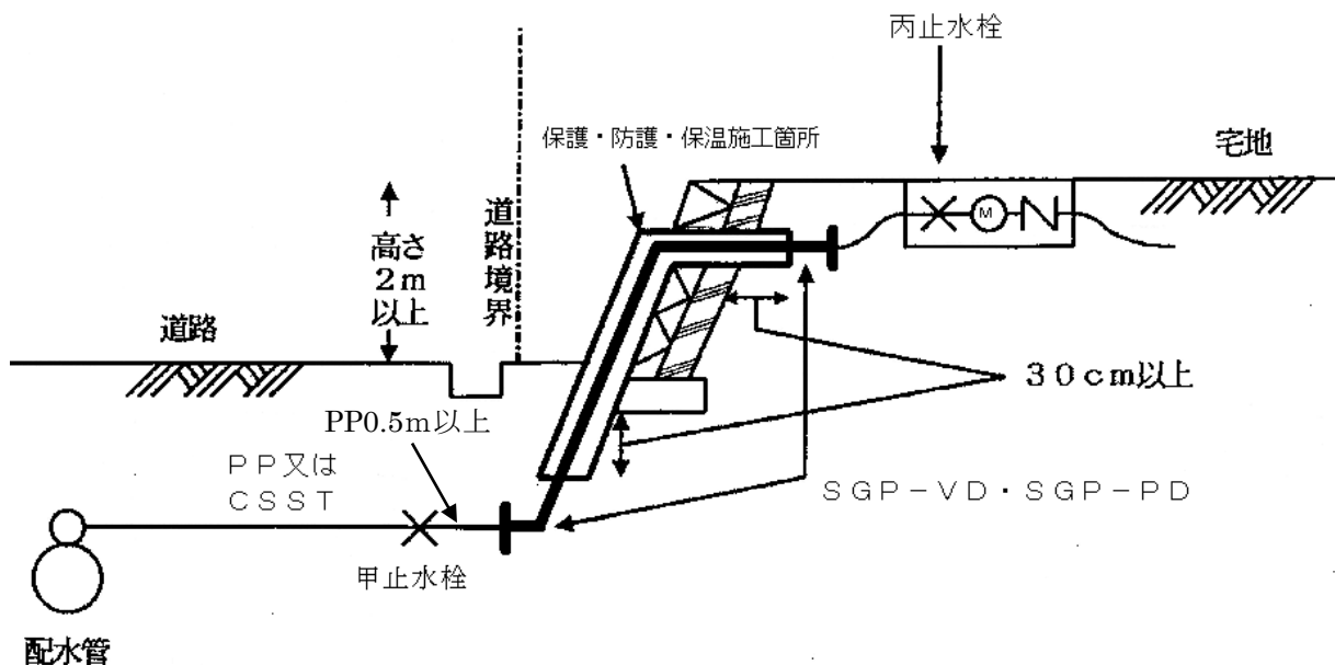
〔石積み及び擁壁露出標準配管図〕 例：φ50 以下の場合
