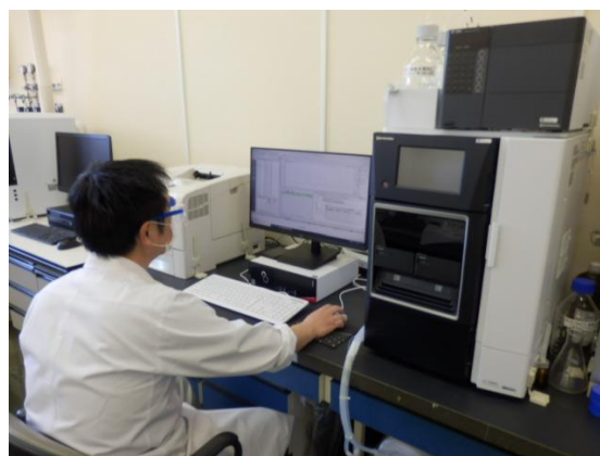
陰イオン界面活性剤を測定している様子 （高速液体クロマトグラフ）
