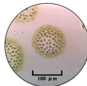
*3 ウログレナ： 黄金藻類の1種で、細胞は楕円形か倒卵形で直径50~200μmの群体をつくる。各細胞先端には長さの異なる2本の鞭毛があり、群体は回転しながら活発に遊泳する。生ぐさ臭を発生する原因として、代表的な生物である。
