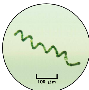
*2 アナベナ： 藍藻類の1種で、糸状体は栄養細胞、異質細胞、休眠胞子で形成されており、らせん状（写真参照）、真っ直ぐ、半円形などの種類が見られる。糸状体の長さは種類によって異なる。
